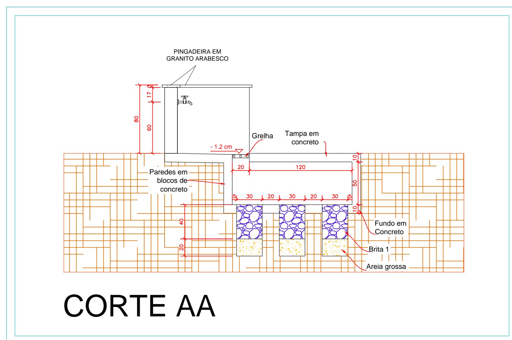
Detalhe 03 - LAVA BOTAS Escala 1:25
